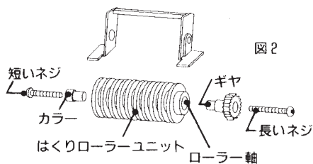
はくりローラー・ホルダーユニット
